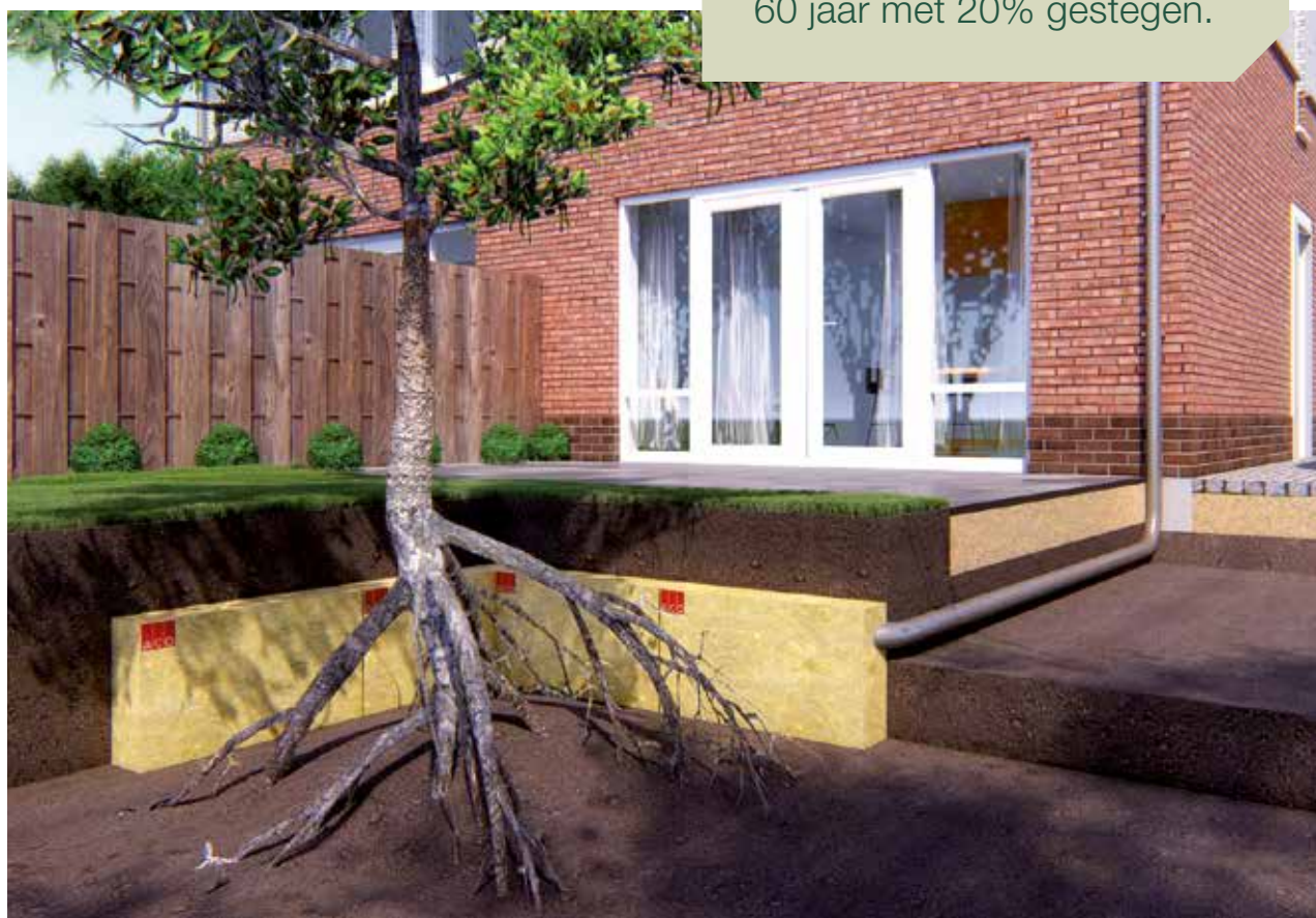
Het duurzame RainBloxx infiltratiesysteem
