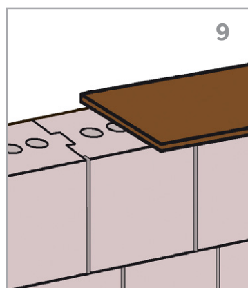
9 Afdekken tijdens onderbreking
