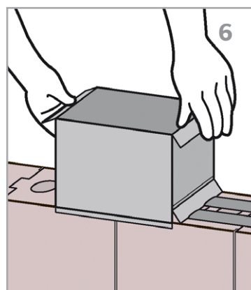
6 Lijm aanbrengen met lijmverdeelbak
