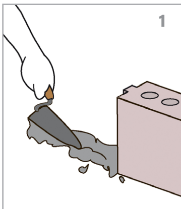
1 Kimblok zetten
