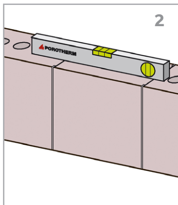
2 Kim waterpas stellen
