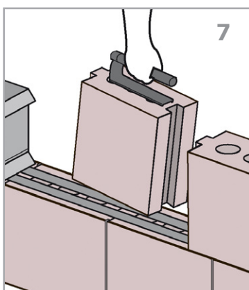
7 Plaatsen lijmblok
