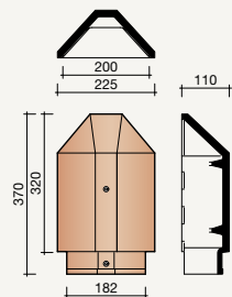
2860 Hoekige beginkepervorst
