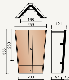
1900 Hoekige schubvorst
