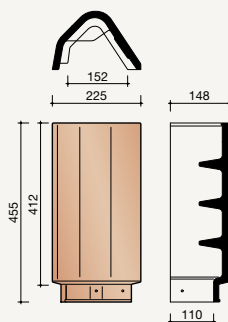
2200 Chaperonvorst*
