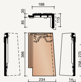
7090 Rechter gevelpan
