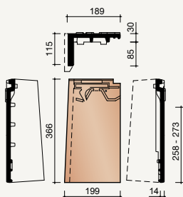
7080 Linker gevelpan
