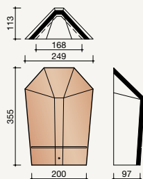
1960 Hoekige beginvorst
