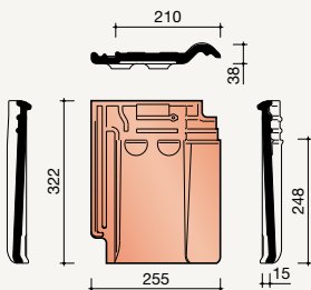
8610 Ventilatie-/haakdoorvoerpan met rooster 12 cm 2
