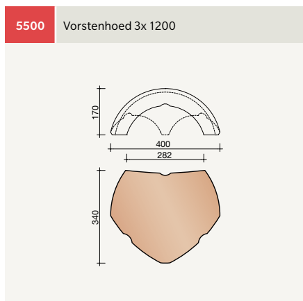
verbindingstuk tussen 3 vorsten
