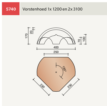
verbindingstuk tussen 2 vorsten en 1 hoekkeper
