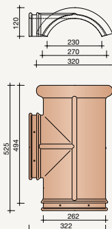
5020 Verbindingsstuk 3x 1200
