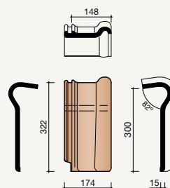
8530 Driekwart chaperonpan
