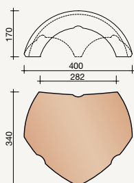
5500 Vorstenhoed 3x 1200
