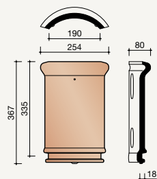
3100 Halfronde hoekkepervorst
