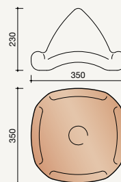
5630 Vorstenhoed 4x 3100
