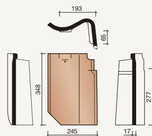
7090 Rechter gevelpan
