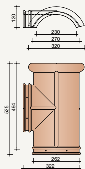
5020 Verbindingsstuk 3 x 1200
