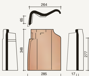
7080 Linker gevelpan
