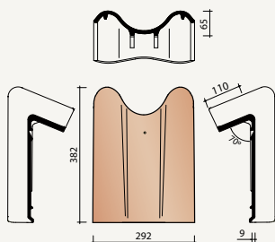
8550 Chaperonpan met dubbele wel
