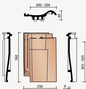
8640 Ventilatie-/haakdoorvoerpan met rooster 28 cm 2
