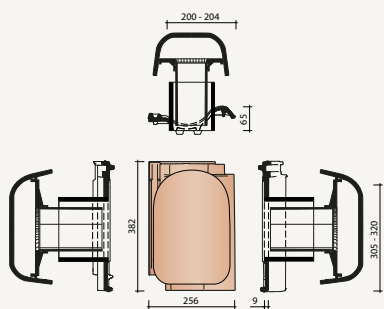
8728 Dakdoorvoer incl. aansl. Ø125 mm
