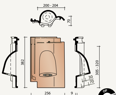
8958 Kabeldoorvoerpan met neopreen ring
