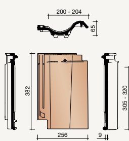
0000 OVH Vario dakpan
