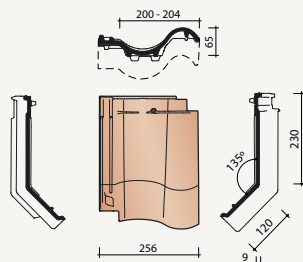
8200 Knikpan op maat (verlijmd)*
