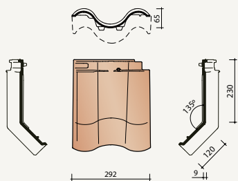
8250 Knikpan met dubbele wel
