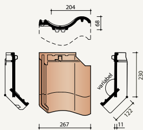
8200 Knikpan op maat (verlijmd)*
