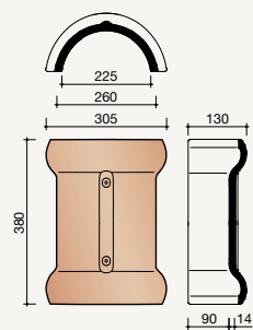
1250 Halfronde vorst met dubbele wel vario
