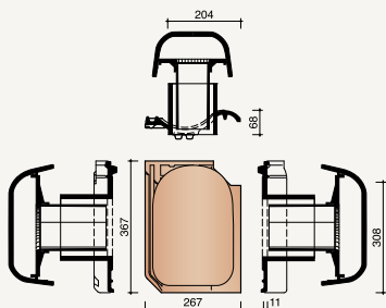
8728 Dakdoorvoer incl. aansl. Ø 125 mm
