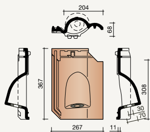
8958 Kabeldoorvoerpan met neopreen ring
