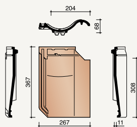
8640 Ventilatie-/haakdoorvoerpan met rooster 25 cm 2
