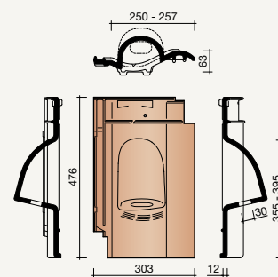
8660 Gierzwaluwpan
