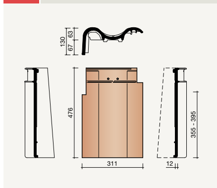
7080 Linker gevelpan
