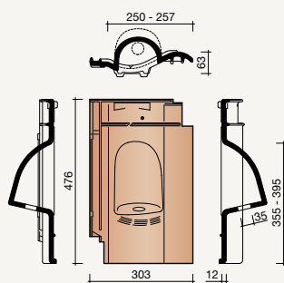
8655 Mussenpan
