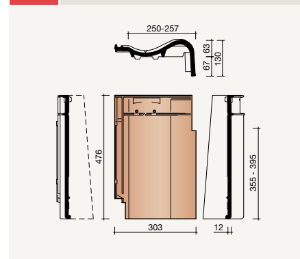
7090 Rechter gevelpan
