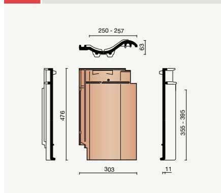
0000 MaduraMax dakpan
