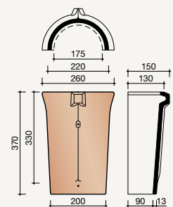
3100 Beginschubvorst
