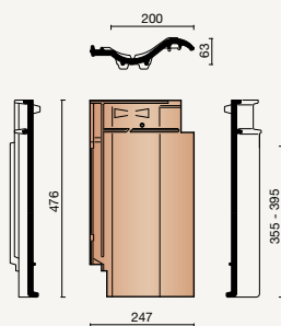
8035 4/5 pan
