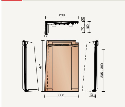
7080 Linker gevelpan
