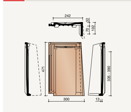
7090 Rechter gevelpan
