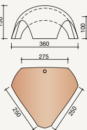
5330 Vorstenhoed 3 x 1001
