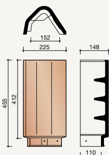
2200 Chaperonvorst
