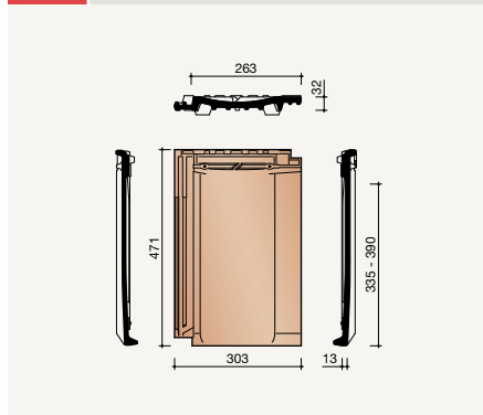
0000 Jura Nova dakpan
