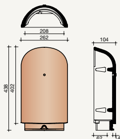
1061 Halfronde beginkeper
