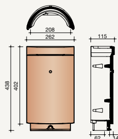
1001 Halfronde vorst
