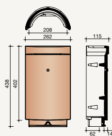
1001 Halfronde vorst
