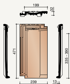
8030 Driekwart pan
