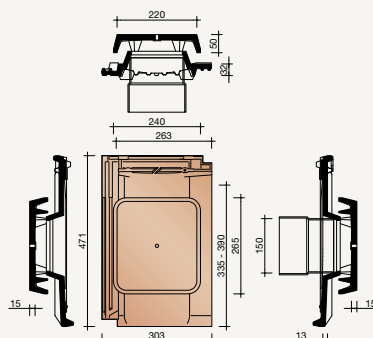
8729 Dakdoorvoerpan Ø 150 mm incl. kapje + aansluitset
