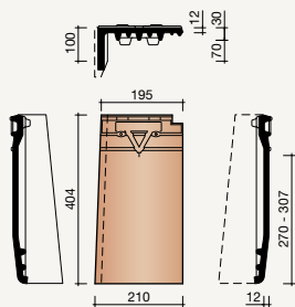
7080 Linker gevelpan
