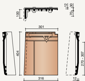
7880 Linker anderhalve gevelpan
