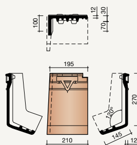
7280 Linker gevelknikpan
