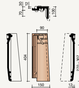
7030 Rechter halve gevelpan
