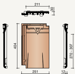
8640 Ventilatie-/haakdoorvoerpan met rooster 26 cm 2
