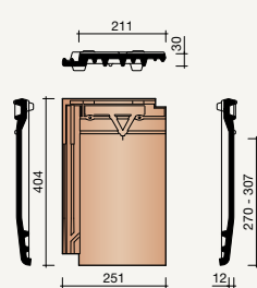
0000 Datura dakpan
