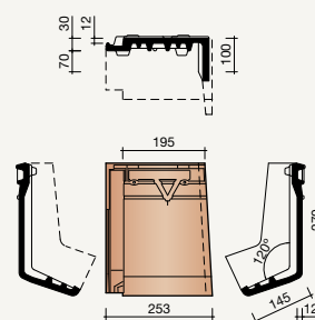
7290 Rechter gevelknikpan
