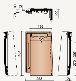
7090 Rechter gevelpan
