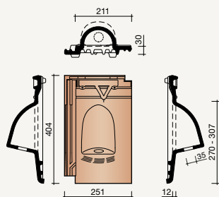
8655 Mussenpan
