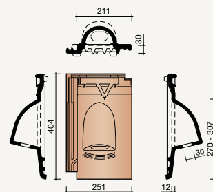
8660 Gierzwaluwp
