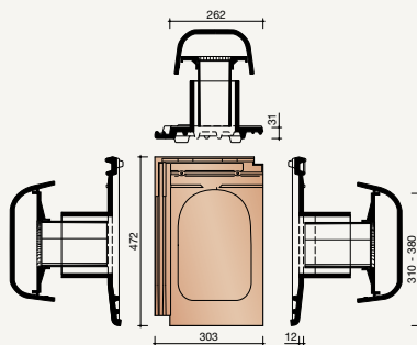
8728 Dakdoorvoerpan incl. aansl. Ø 125 mm
