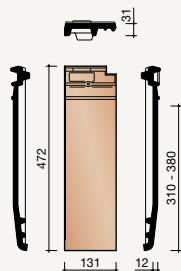
8040 Halve pan zonder zijsluiting
