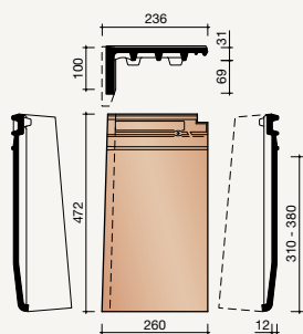
7080 Linker gevelpan
