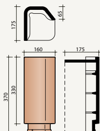
4930 Begin chaperonvorst
