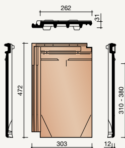
8640 Ventilatie-/haakdoorvoerpan met rooster 26 cm 2
