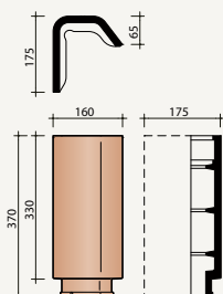
4900 Chaperonvorst
