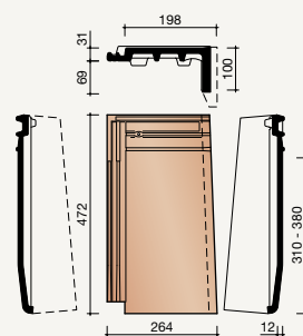
7090 Rechter gevelpan
