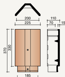
2800 Hoekige vorst
