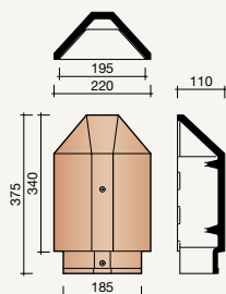
2860 Hoekige beginkepervorst
