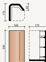
4920 Eind chaperonvorst
