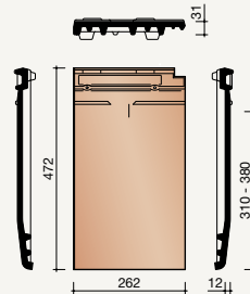
8045 Pan zonder zijsluiting
