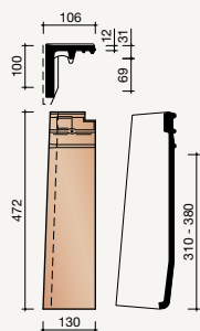
7020 Linker halve gevelpan
