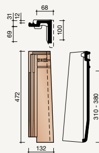
7030 Rechter halve gevelpan
