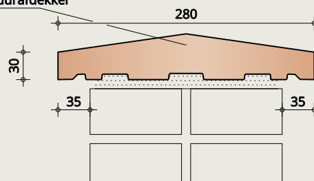
keramische muurafdekker
