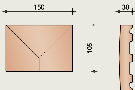
keramische muurafdekker
