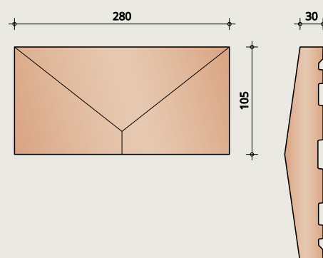
keramische muurafdekker
