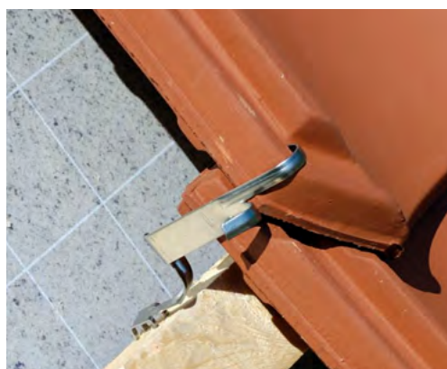
Veilig verankeren: voor elk dakpanmodel is er een geschikte panhaak.
