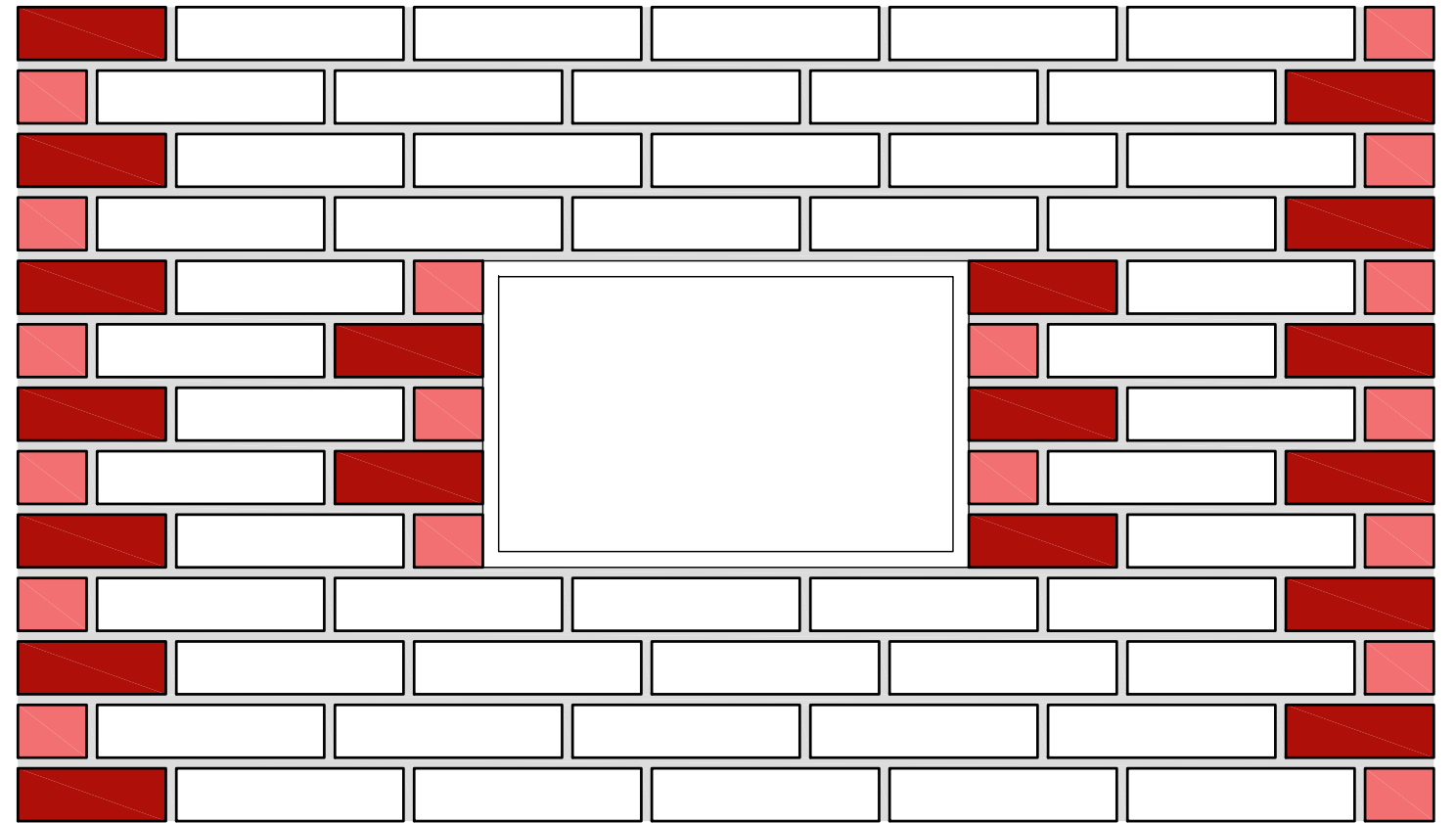
VOORAANZICHT
