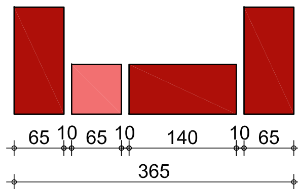
LAAG 1
