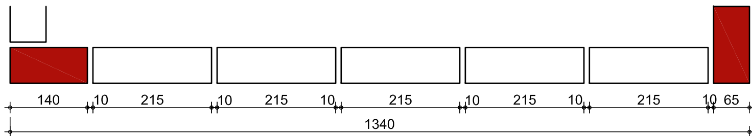
PLATTEGROND
