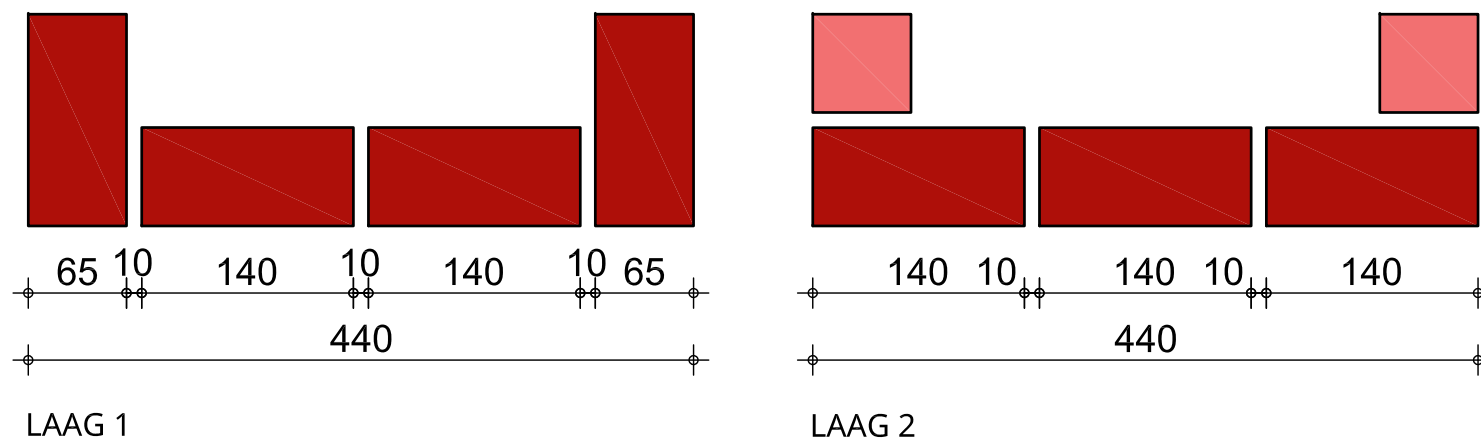
PLATTEGROND
