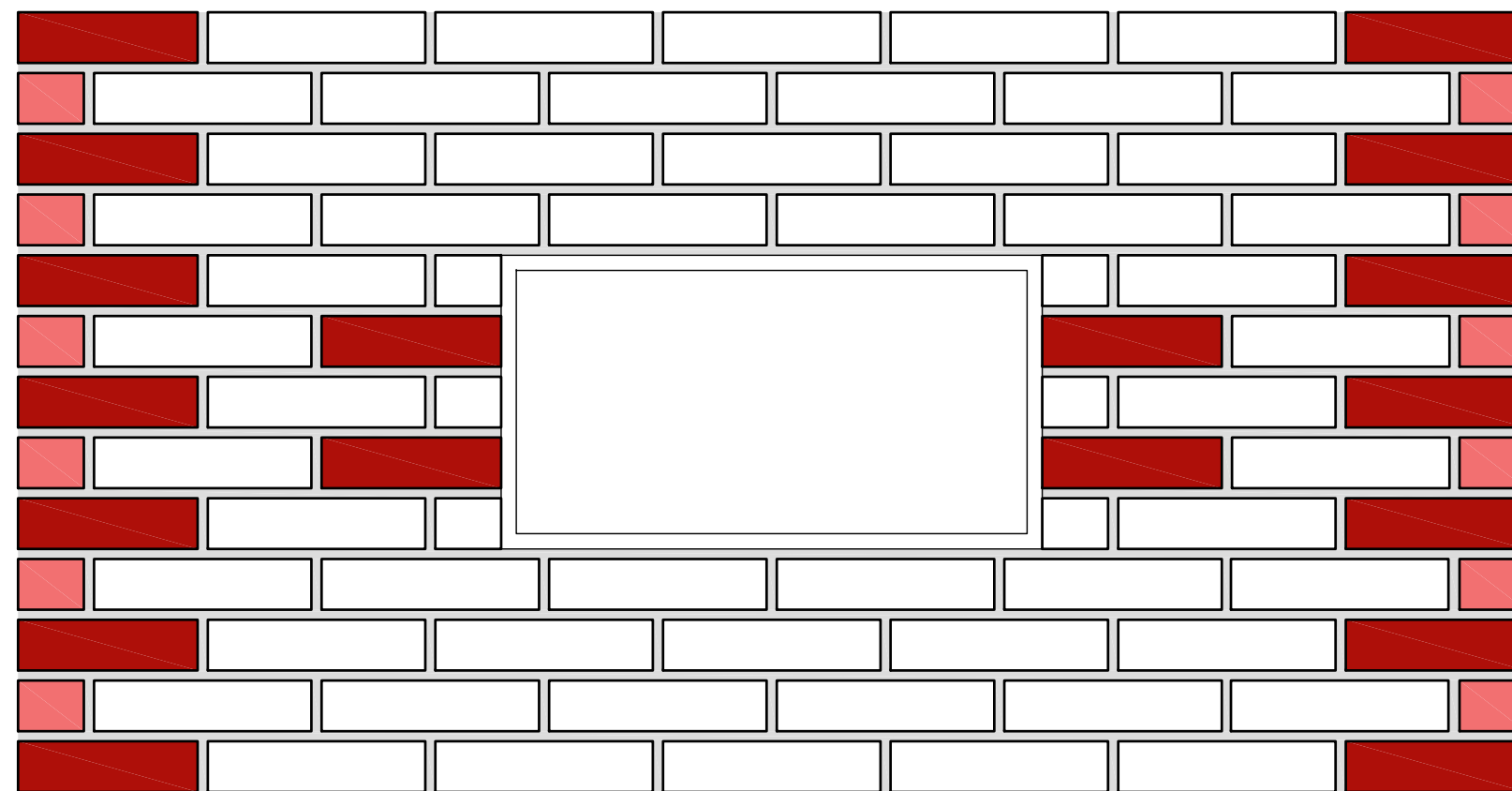
VOORAANZICHT
