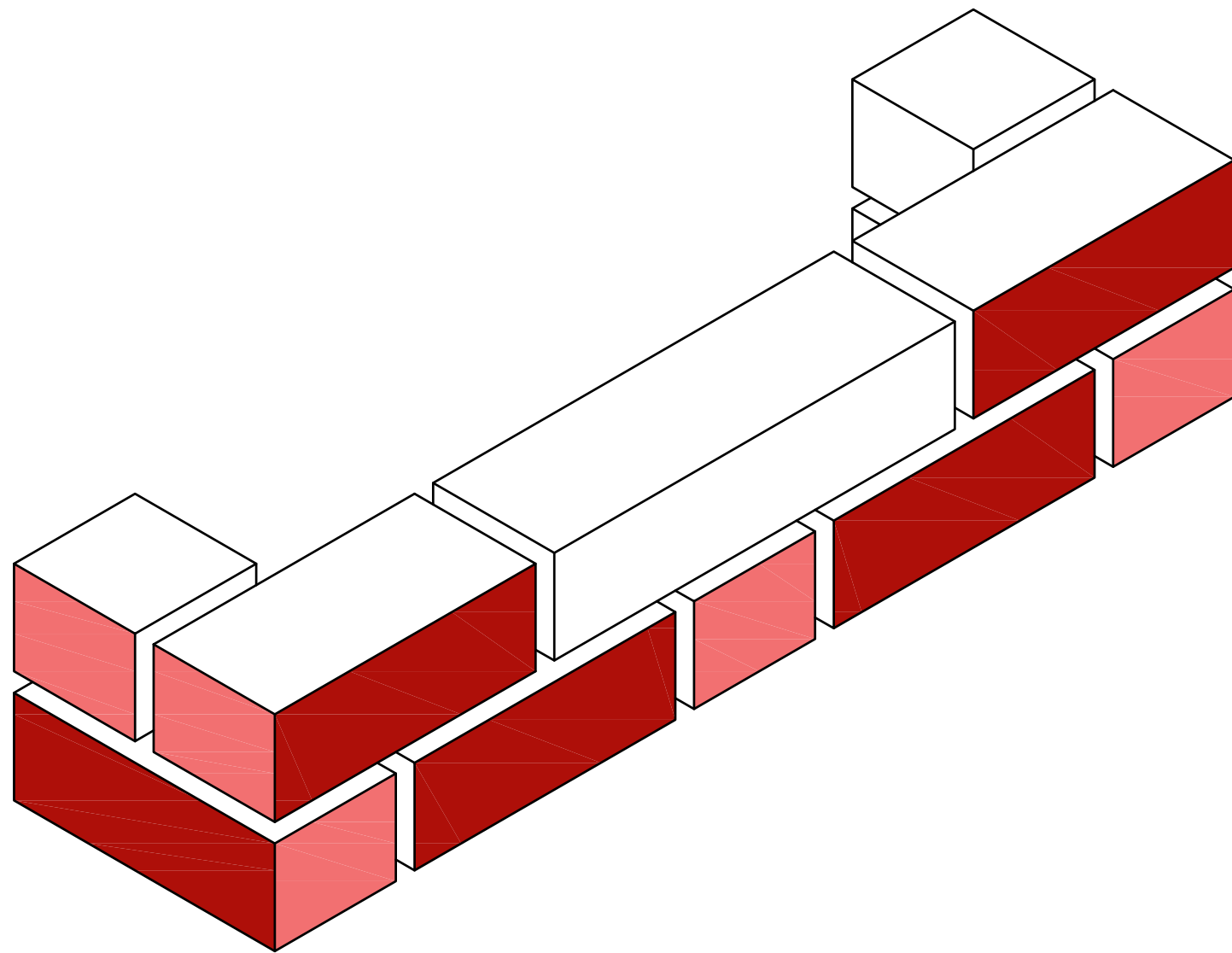
3D AANZICHT
