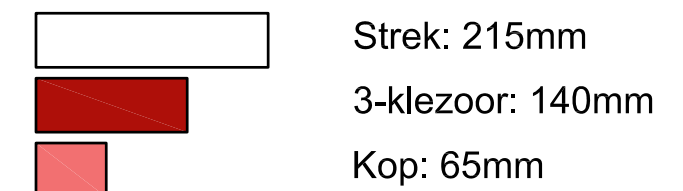
MAATVOERING
