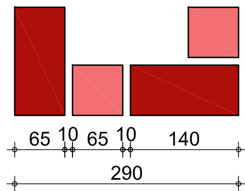
LAAG 1
