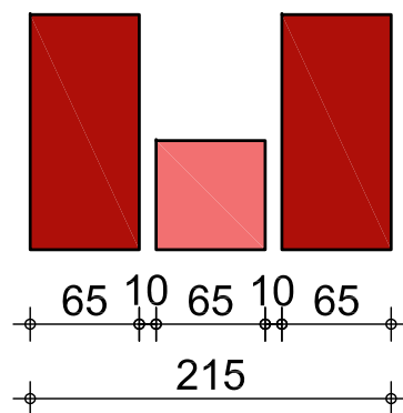
LAAG 1
